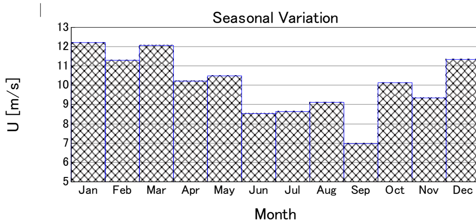
図 4-1-2 月平均風速の季節変化（龍飛埼灯台、1997年）
