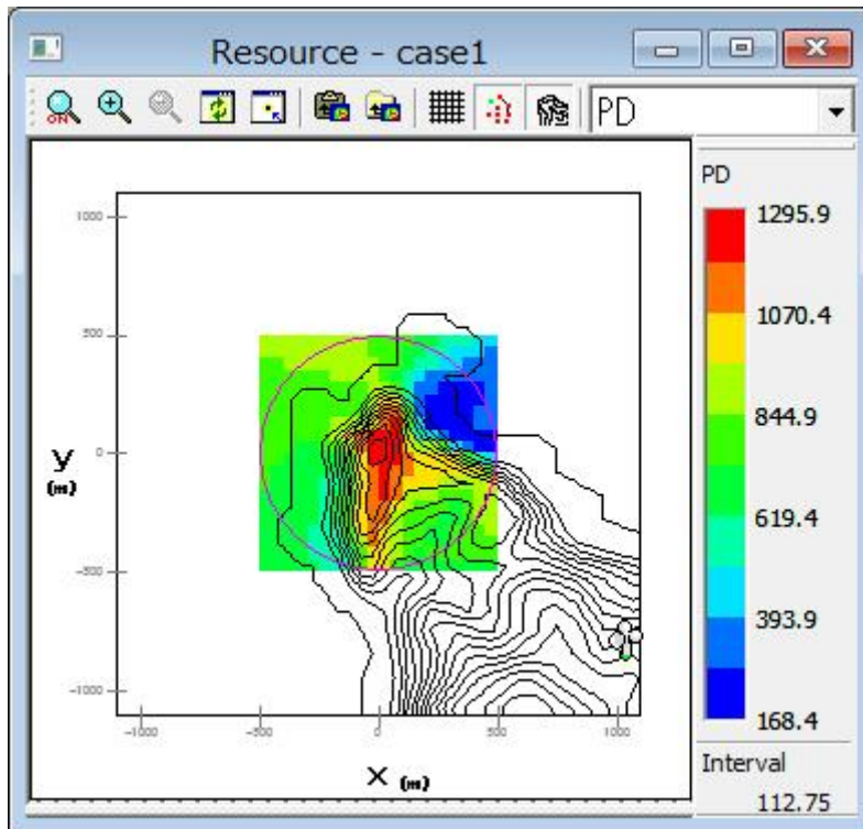
例 4：風力エネルギー密度分布図 [PD]
