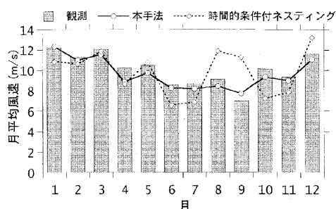
図-22 龍飛崎灯台における月平均風速
