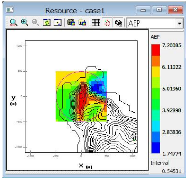
例 5 : 年間発電量分布図 [AEP]
