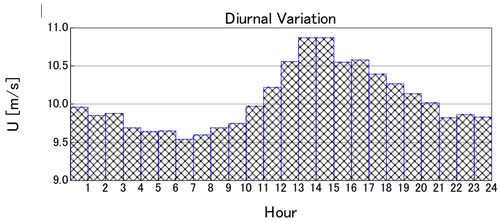
図 4-1-1 時間平均風速の日変化（龍飛埼灯台、1997年）
