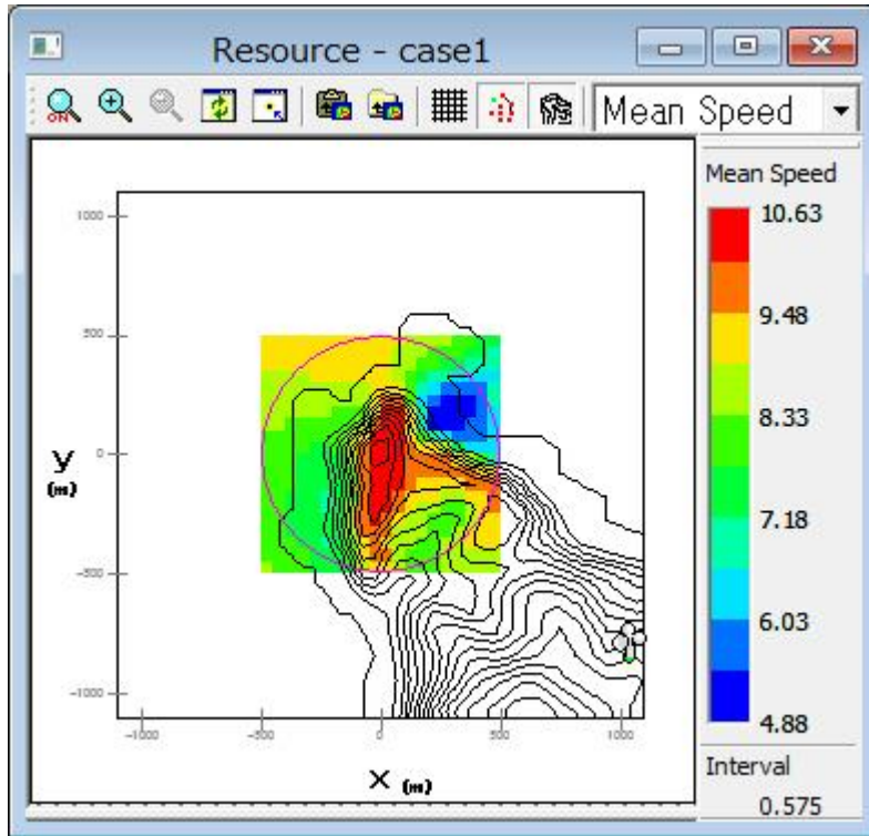
例 3：平均風速分布図 [Mean Speed]
