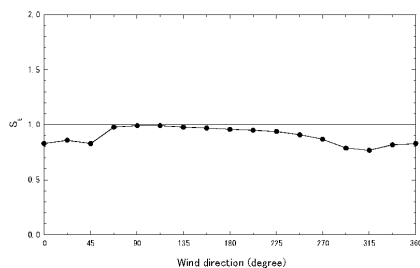
図 11 平均風速の割増係数の風向による変化 (Variation of speed-up ratio of mean wind speed with wind direction)
