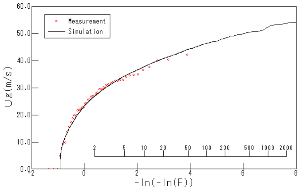
図 - 4.4 上空風の年最大風速の例
