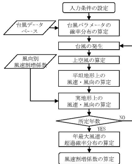
図1 風速割増係数算定の手順
