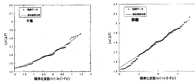
図 2 気圧低下量の混合確率分布関数による近似
