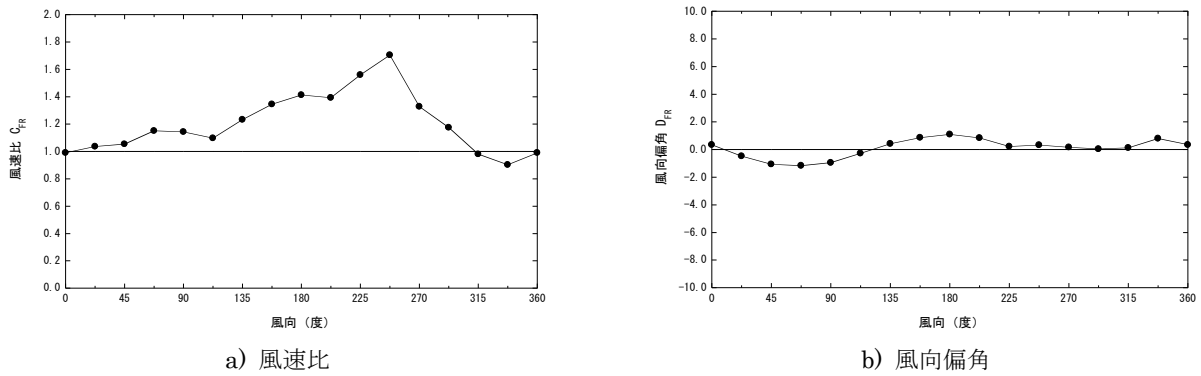
図 - 4.6 気流解析からより求めた風速比および風向偏差の風向変化
