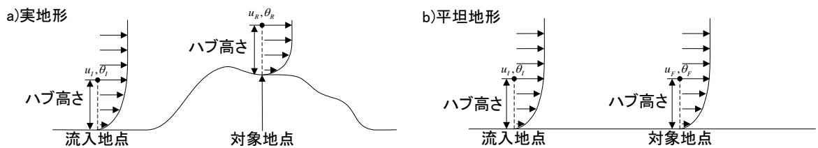
図 - 4.5 実地形上と平坦地形上における気流解析の模式図
