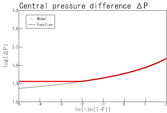
a) 中心気圧低下量 \Delta P
