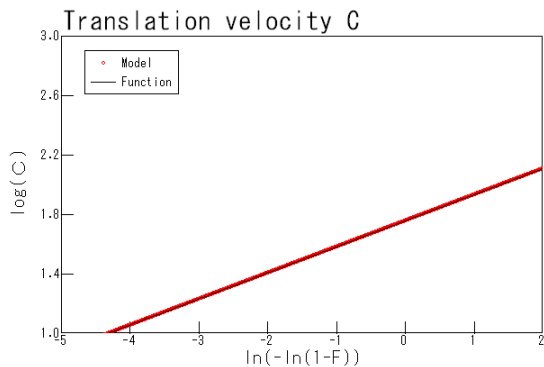
c) 進行速度 C
