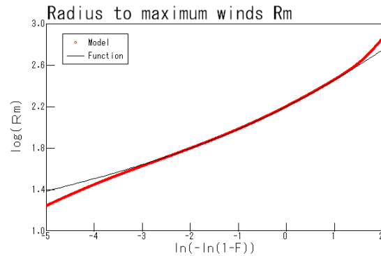
b) 最大旋衡風速半径 R_m
