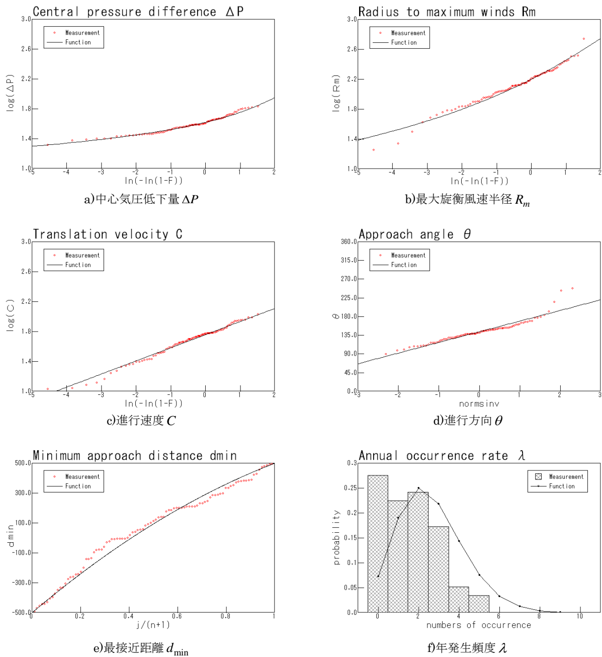
図 - 4.2 台風パラメータの確率分布の例
