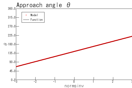
d) 進行方向 \theta
