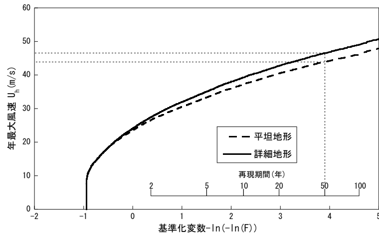
図 - 4.7 平坦地形と実地形上の台風による年最大風速の非超過確率分布の例
