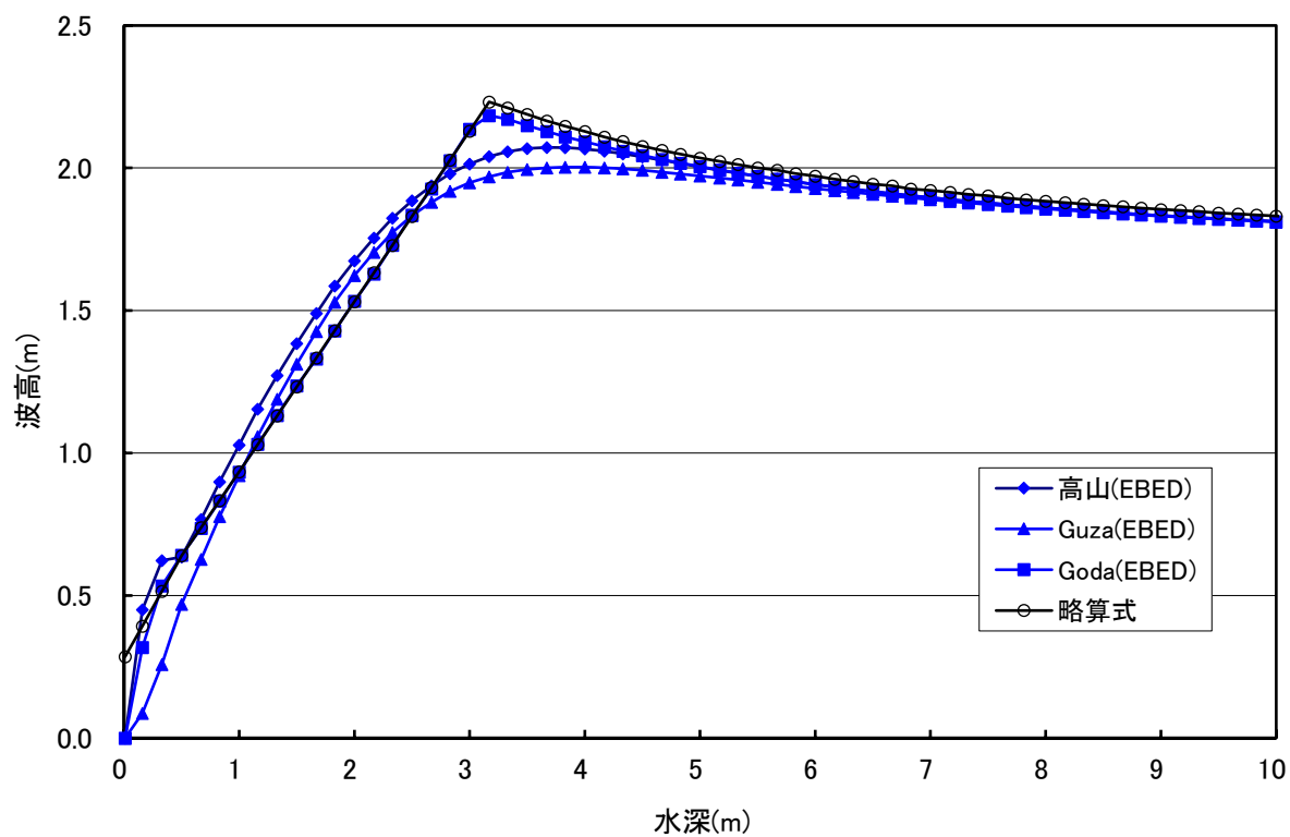
図- 3-2.3 碎波計算の比較
