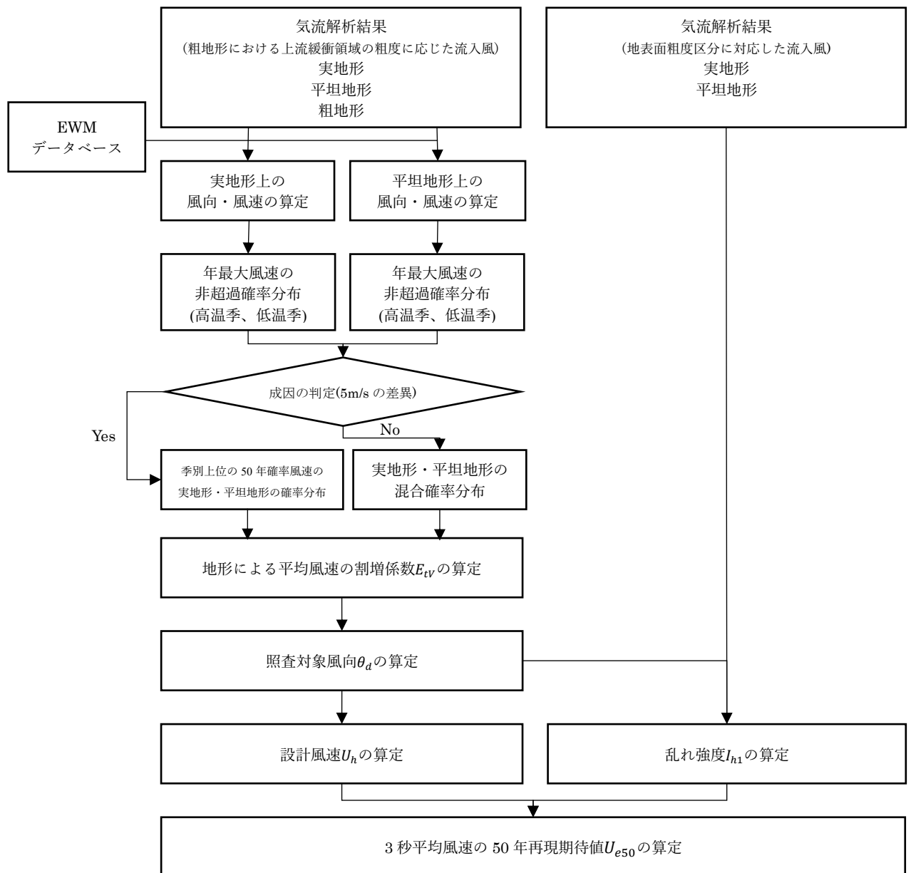
図 - 3.1 設計風速算定のフロー
