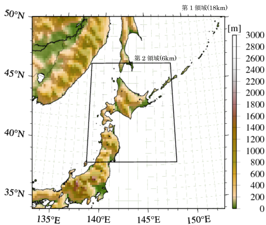
図 - 3.2 WRF の解析領域
