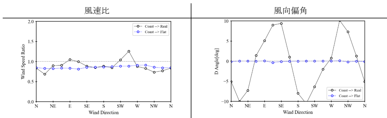
図 - 3.3 風速比、風向偏角の例
